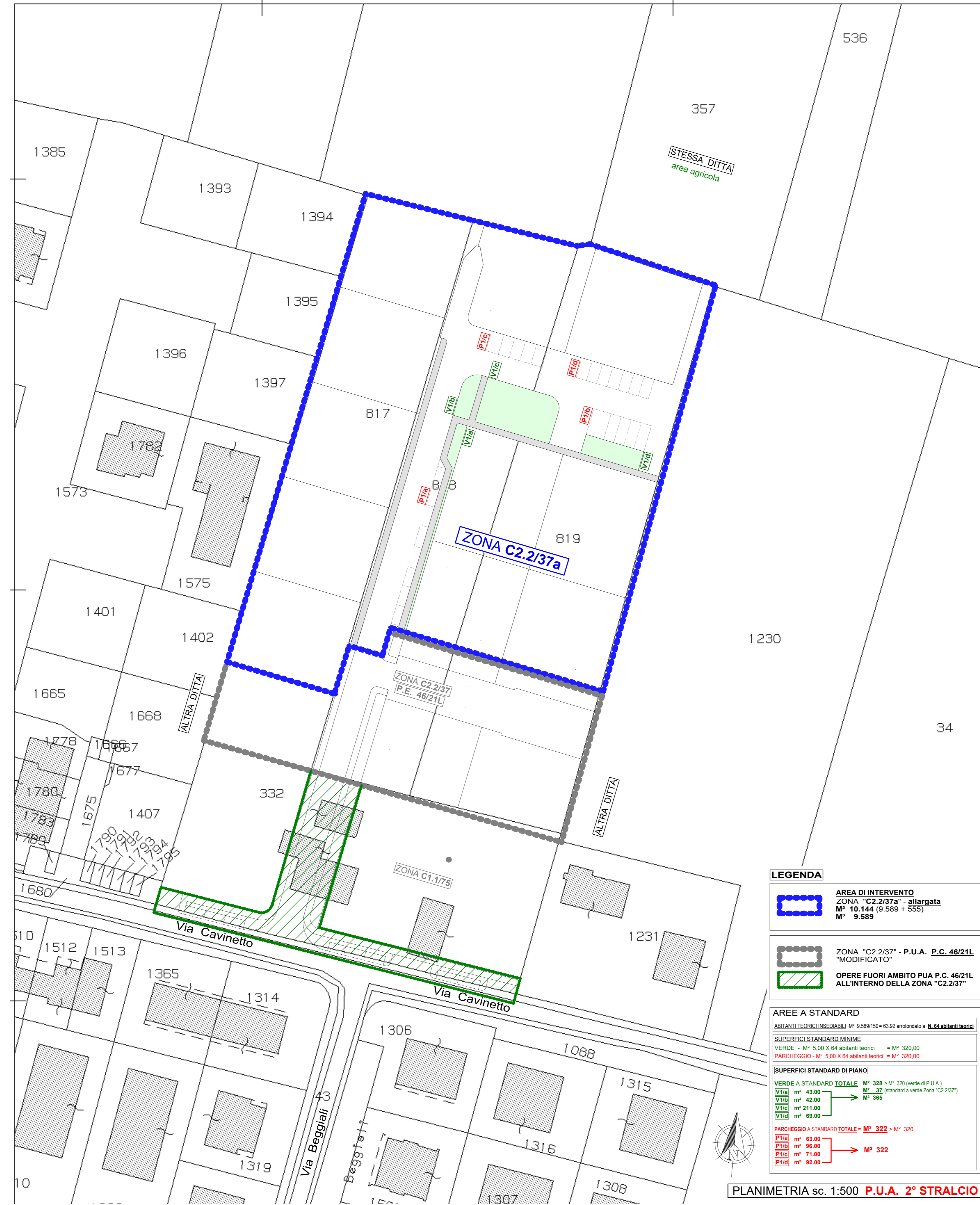
PLANIMETRIA PROGETTO PUA - 2° STRALCIO
